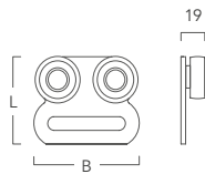
Nylonrolle Ø 32 mm Trike VS mit Schlitz
