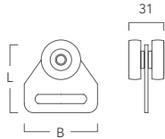
Nylonrolle Ø 32 mm mit Schlitz
