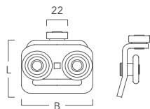
Doppelrolle Nylon Ø 31 mm gekröpft mit Kugellager
